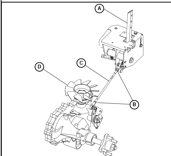
A. Steering control lever B. Jam nuts
